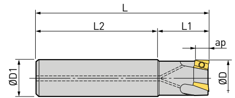
Fresatura a spallamento
